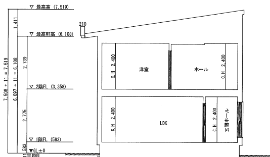
Y-Y' 断面図 S=1/100
